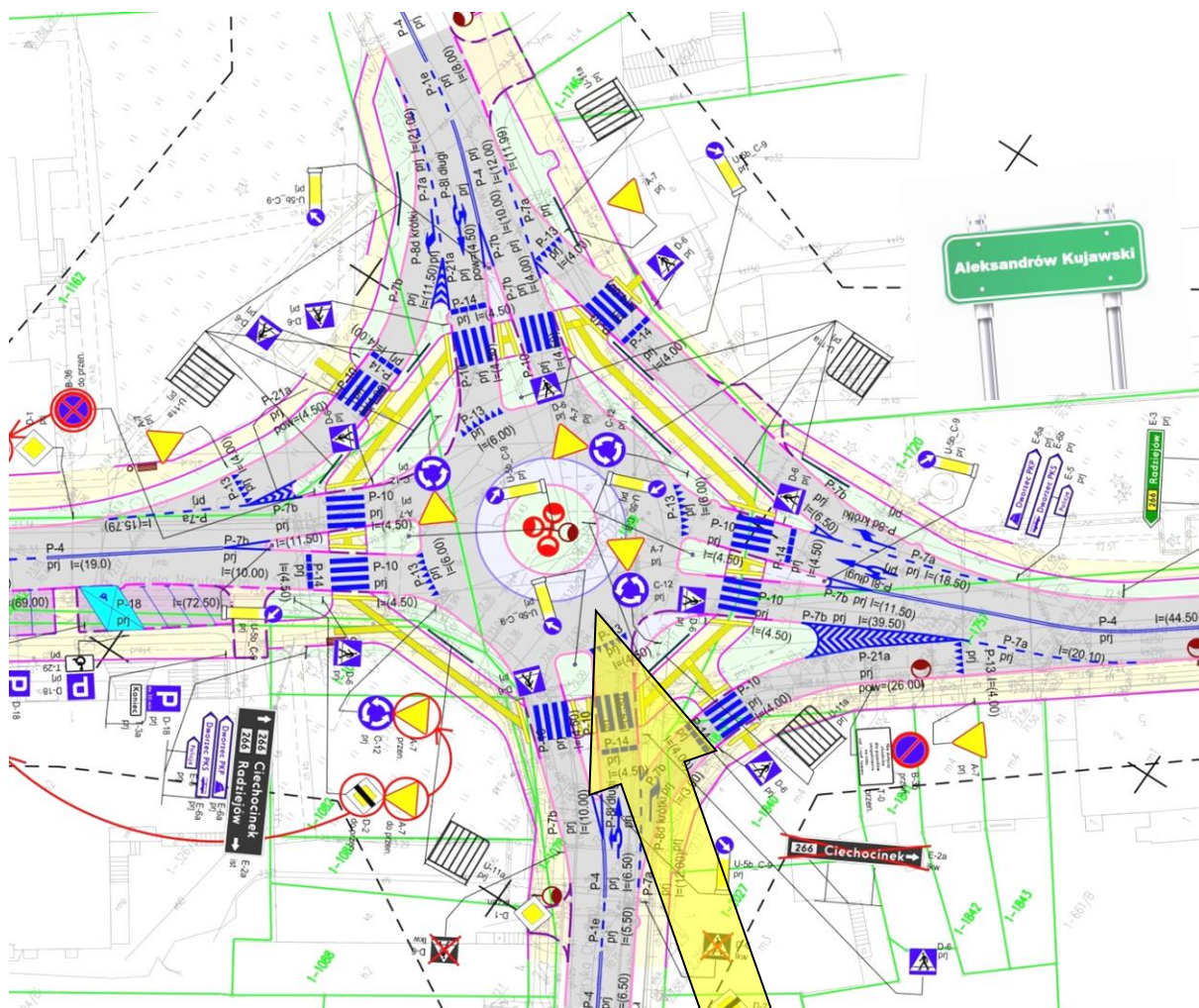
Ryc 3. Projekt stałej organizacji ruchu na budowanym w Aleksandrowie Kujawskim rondzie – skrzyżowanie ulic: Słowackiego, Dworcowa, Narutowicza, Chopina.
