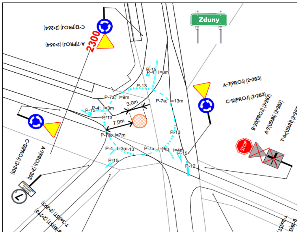
Ryc. 1. Projekt SOR dla skrzyżowania DP 2530C w miejscowości Zduny.
