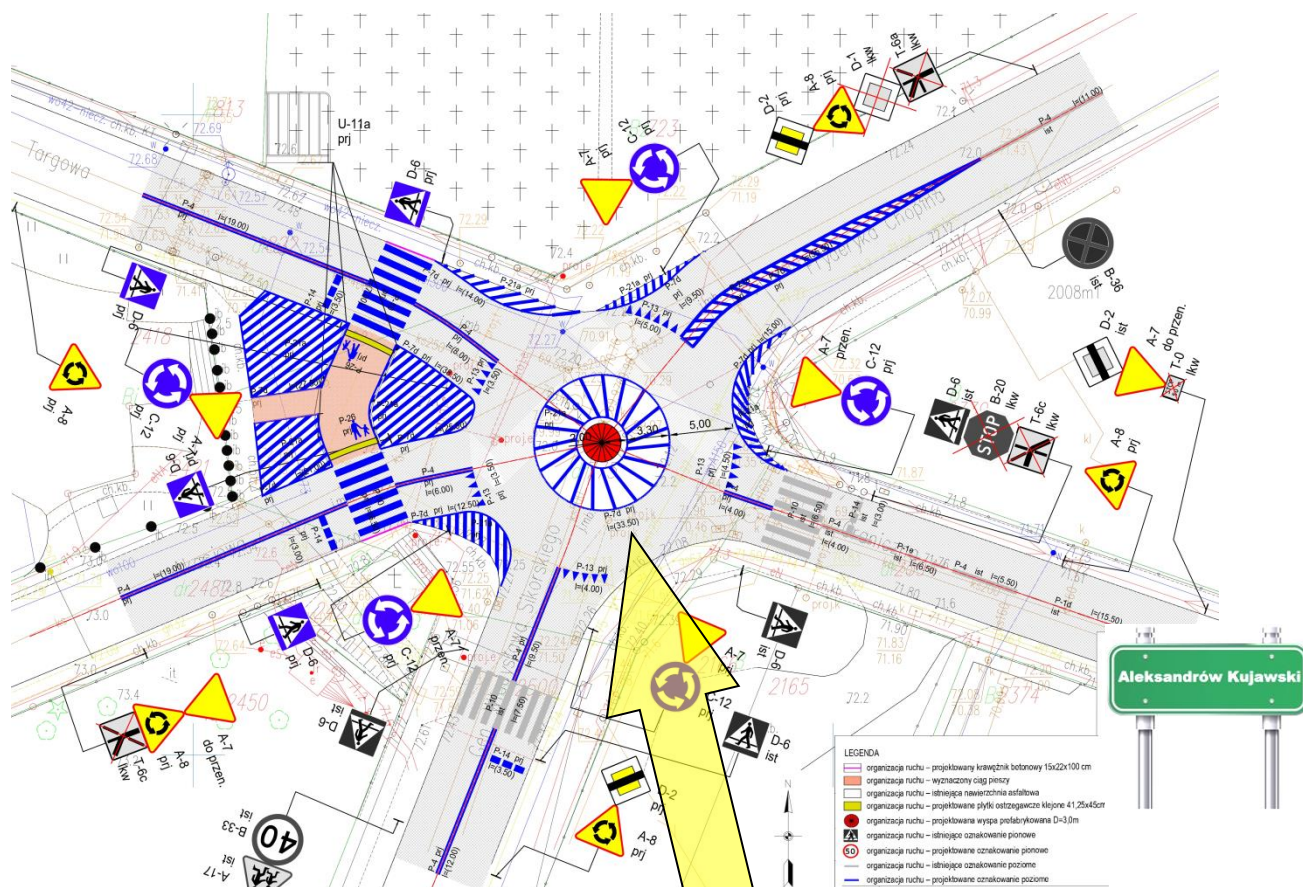
Ryc. 2. Projekt SOR dla skrzyżowania DP 2632C z ul.: Chopina, Sikorskiego, Akacyjowa i Targowa.
