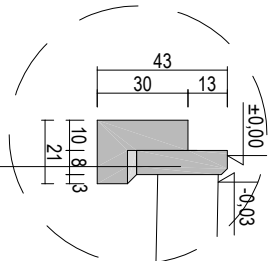
SZCZEGÓŁ "B"
