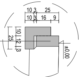
SZCZEGÓŁ "D"
