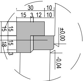
SZCZEGÓŁ "C"
