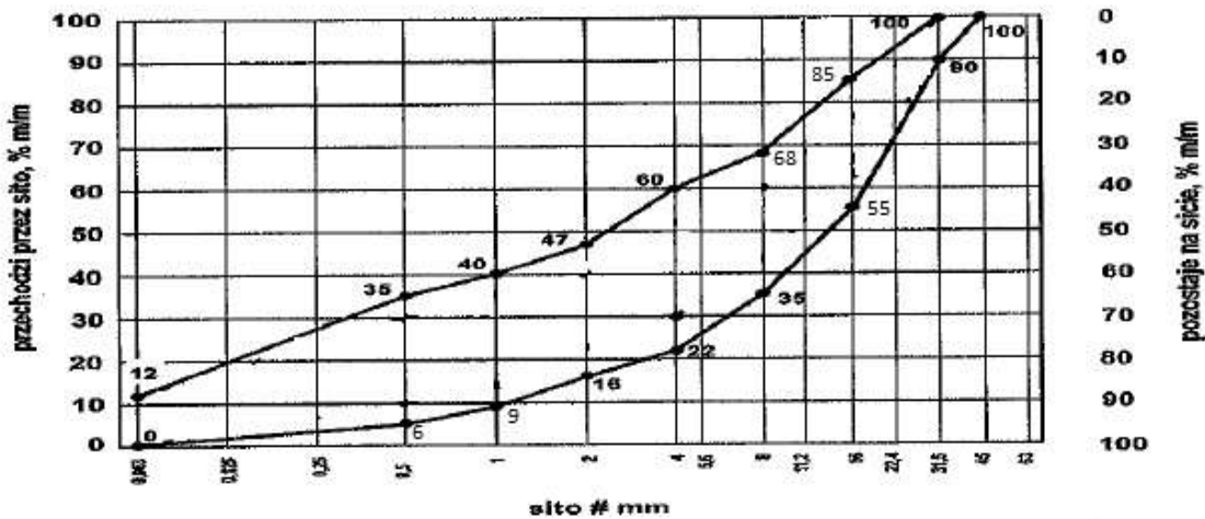
Rysunek 1. Mieszanka niezwiązana 0/31,5 do warstwy ulepszonego podłoża stabilizowanego georusztem 2.4. Parametry mieszanki niezwiązanej
