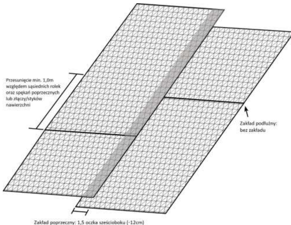
Rys. 1 Szczegół dotyczący wykonania zakładów (zakład poprzeczny tylko w przypadku uszczegółowionych zapisów projektowych – w innym przypadku łączenie sąsiednich rolek ,na styk' lub z minimalnym zakładem)
